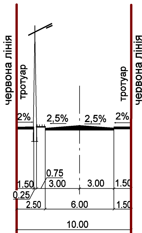
Розріз I-I
